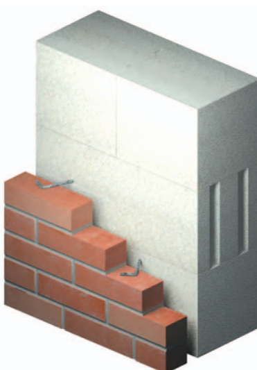
Рис. 7б. Облицовка с непосредственным креплением
