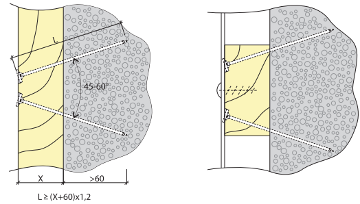
а – деревянный брусок, набитый на кладку непосредственно
