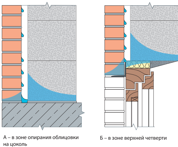
Рис. 8. Конденсат на внутренней поверхности облицовки. Зона потенциального увлажнения
