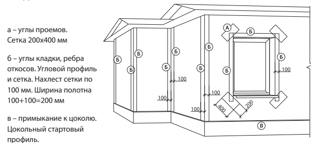
Рис. 15. Схема армирования штукатурки
